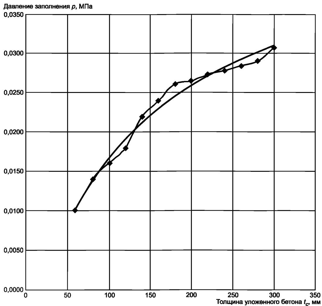
Рисунок Е.1 — Давление на опалубку свежесуложенного бетона
